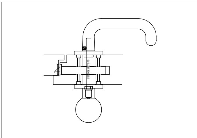
Wechsel- garnitur
