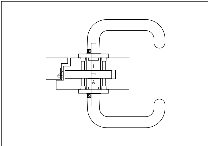
Türdrücker- garnitur
