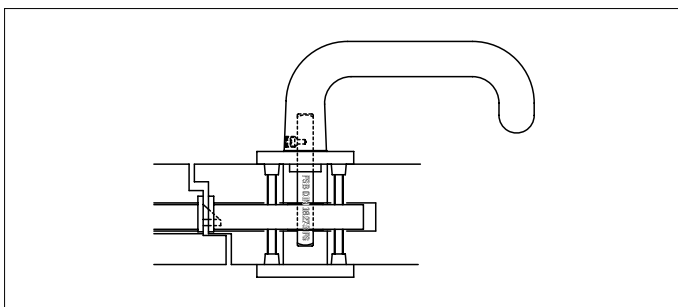
Standflügel- garnitur*
